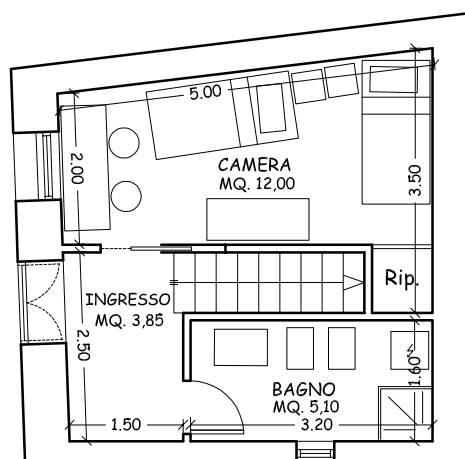
PIANTA PIANO TERRA SUP COMMERCIALE 33,50 MQ
