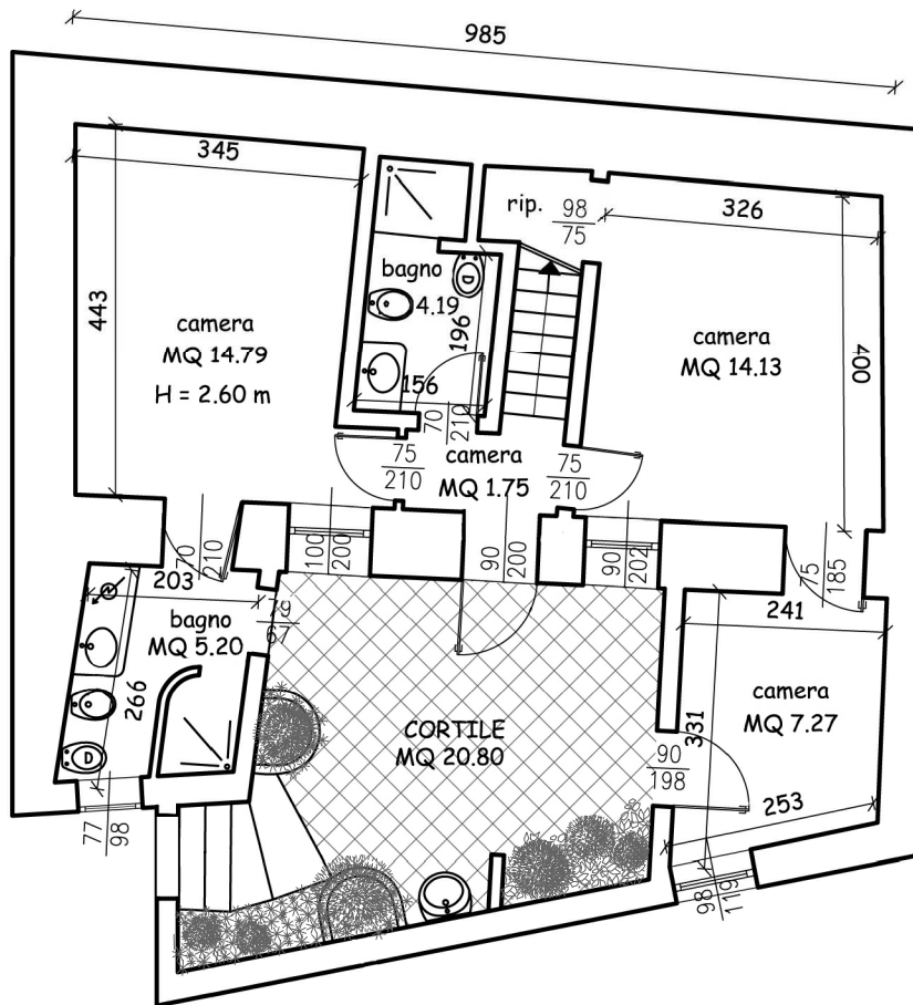
PIANTA PIANO TERRA SUP 77 MQ + CORTILE 21 MQ
